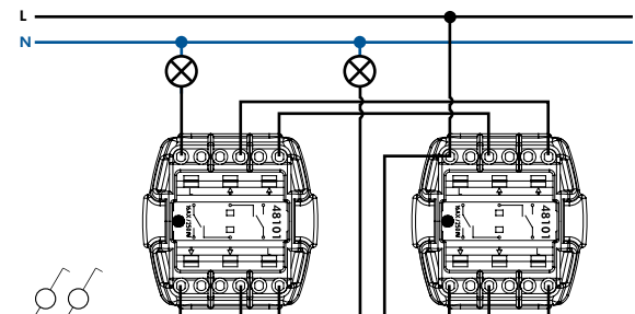
DOBLE CONMUTADOR
