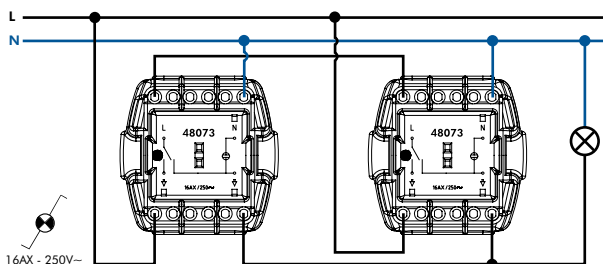
CONMUTADOR CON PILOTO DE SEÑALIZACIÓN
