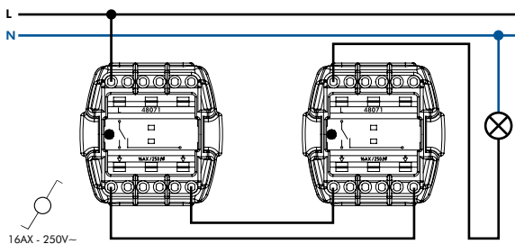
CONMUTADOR
