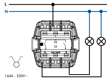
CONMUTADOR LUMINOSO
