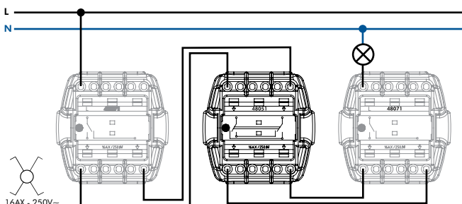
CONMUTADOR DE CRUCE
